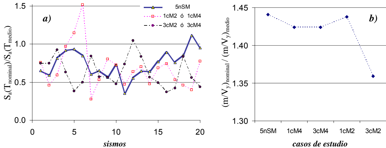
Figura 4.22 Relaciones a) S_a(T_{nominal})/S_a(T_{medio}) y b) (m/V_y)_{nominal} / (m/V_y)_{medio} para los casos de estudio
