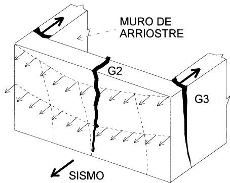
Figura 2. Fallas típicas en viviendas de adobe por acción sísmica perpendicular al plano de los muros: desgarramiento vertical en las esquinas y grieta vertical por flexión en la zona central del muro.
