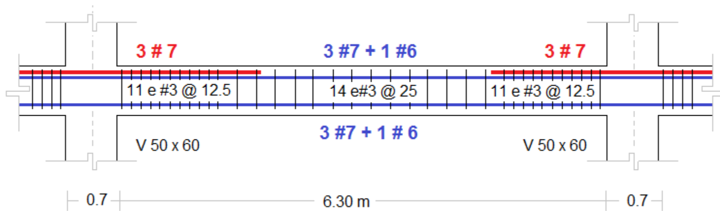
(b) Resistencia a colapso: Env: (a) + Diseño CP: 1.25f'_c , 1.25f_y , \phi=1 , D+0.25L , DMI
