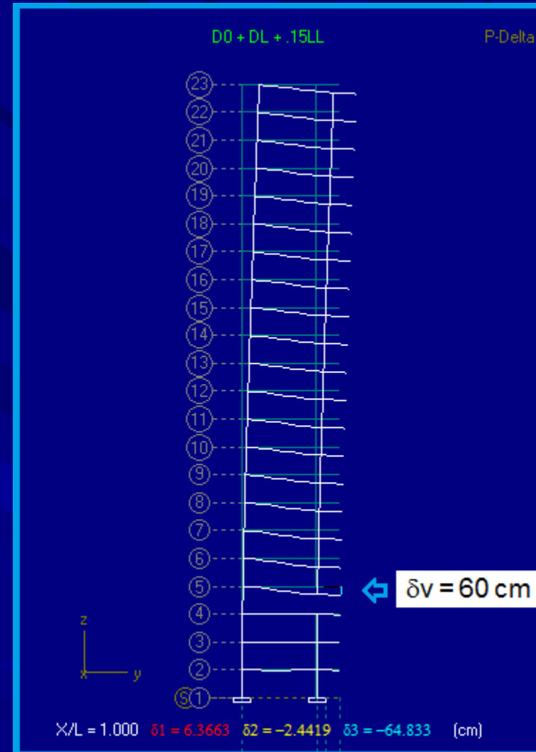
(b) Despues de falla local
