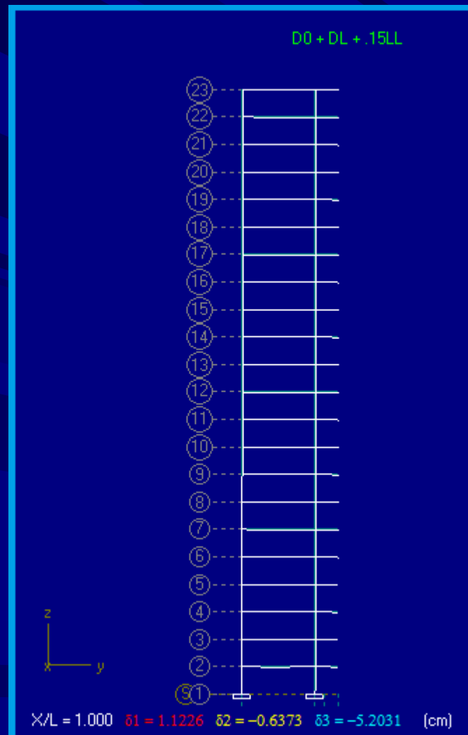
(a) Antes de falla local
