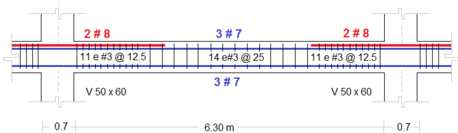
(a) Diseño original: f'_c , f_y , \phi , Envolvente combinaciones de carga, DMO
