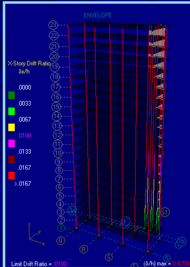
(a) Derivas Dirección X ( \delta/h max = 42%)
