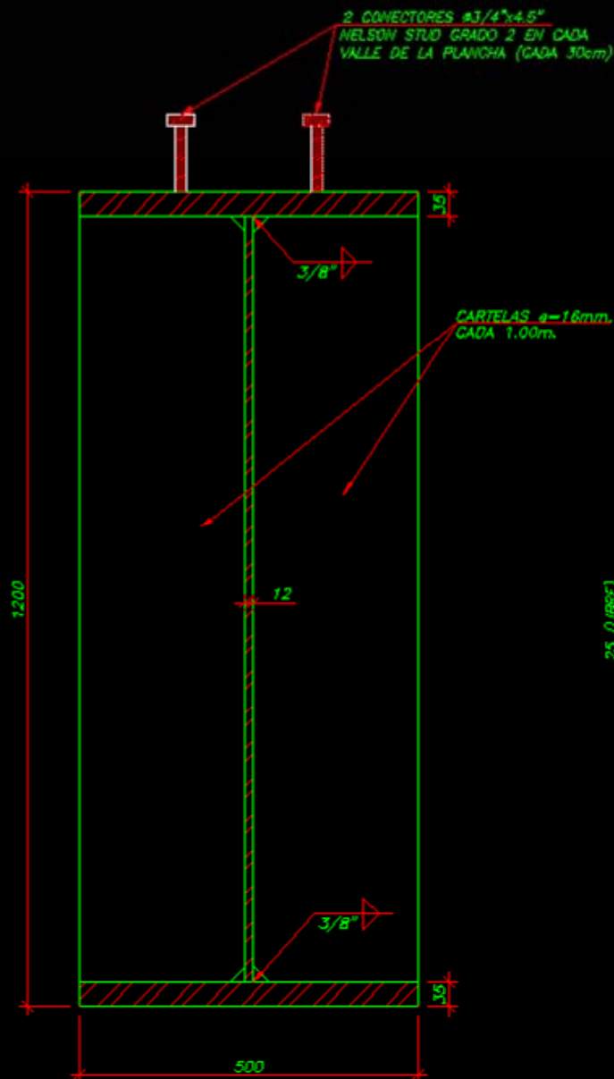
VIGA VM-1 ESCALA: 1/7.5
