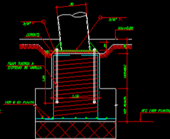
ELEVACION APOYO DE COLUMNA P26
