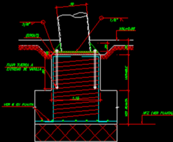
ELEVACION APOYO DE COLUMNA P25
