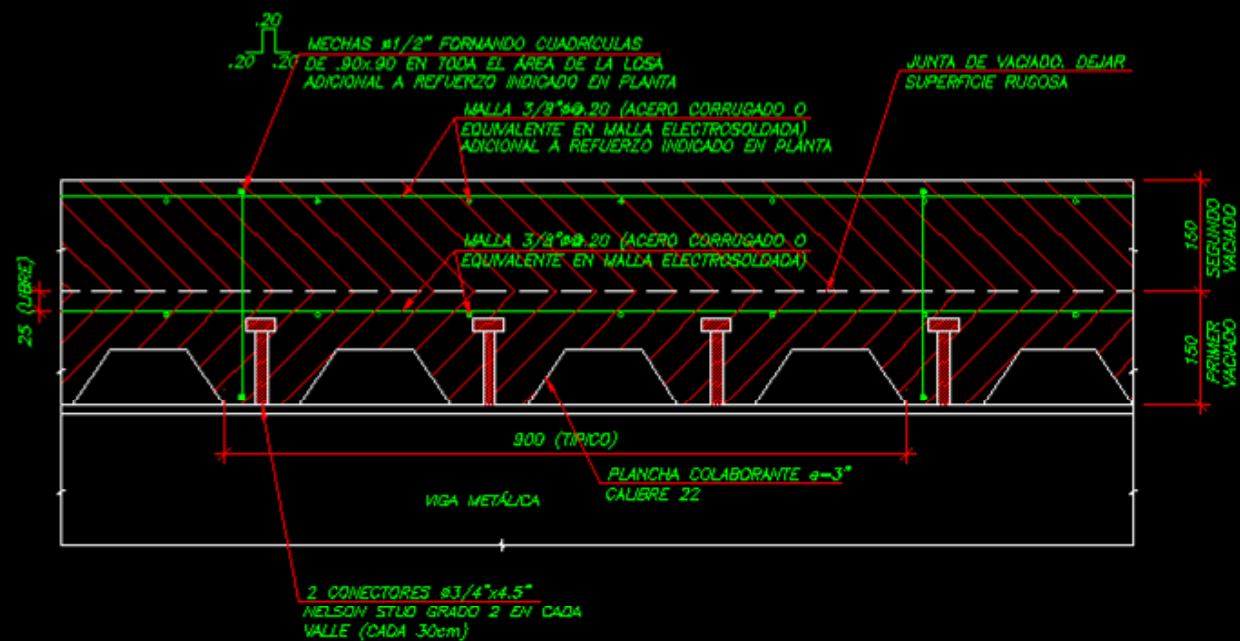
DETALLE DE LOSA CON PLANCHILLA COLABORANTE ESCALA: 1/7.5
