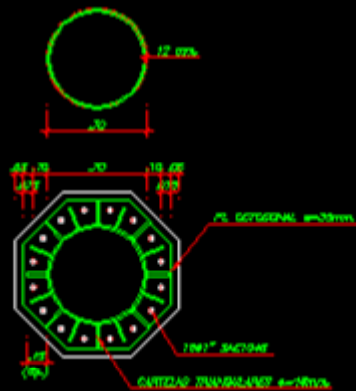
PLANTA PLANCHA BASE
