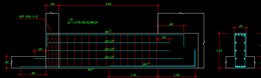
VIGA VC-7 (.40x1.20)
