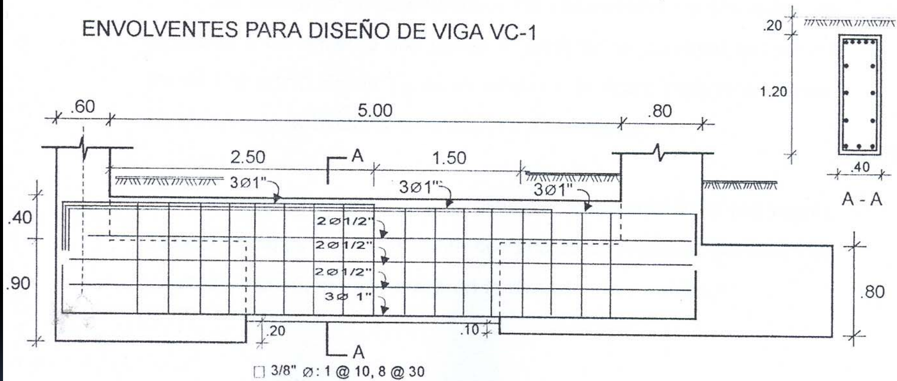
DISEÑO FINAL DE VIGA DE CONEXION VC-1
