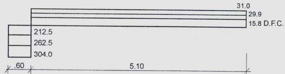
ENVOLVENTES PARA DISEÑO DE VIGA VC-1
