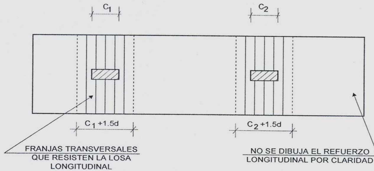
ZAPATA COMBINADA ALARGADA
