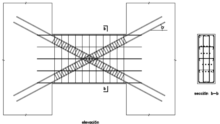
Fig. 21.9.9.5 ii Refuerzo alternativo de vigas de acople.
