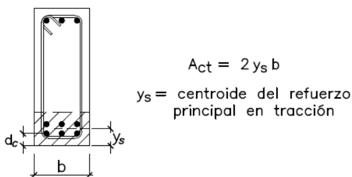
Fig. 9.9.3 Área efectiva de concreto en tracción.
