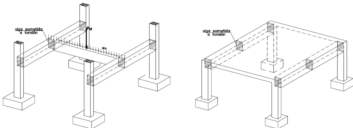
Fig. 11.6.2.2 Casos en los cuales la resistencia a la torsión no afecta directamente al equilibrio de la estructura (torsión de compatibilidad)
