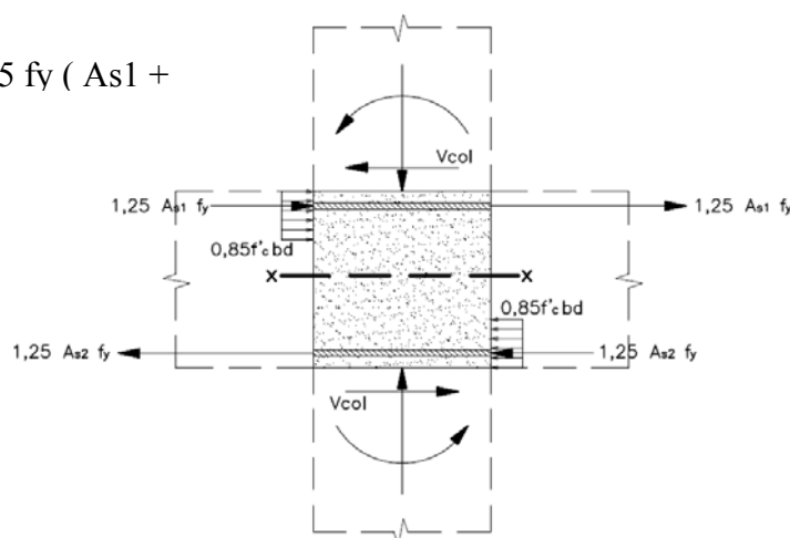
Fig. 21.7.4.3 Fuerzas para el cálculo del cortante en el nudo.
