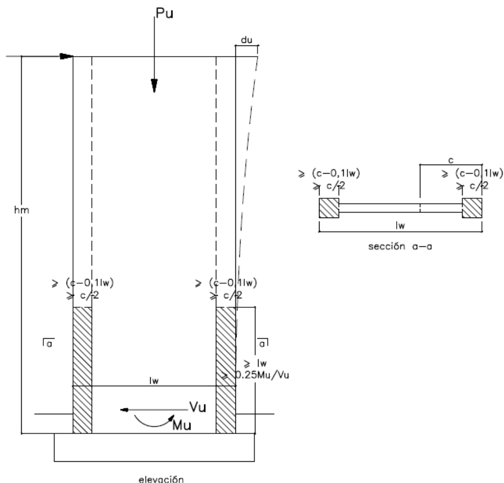
Fig. 21.9.7.4 Elementos confinados de borde en muros.
