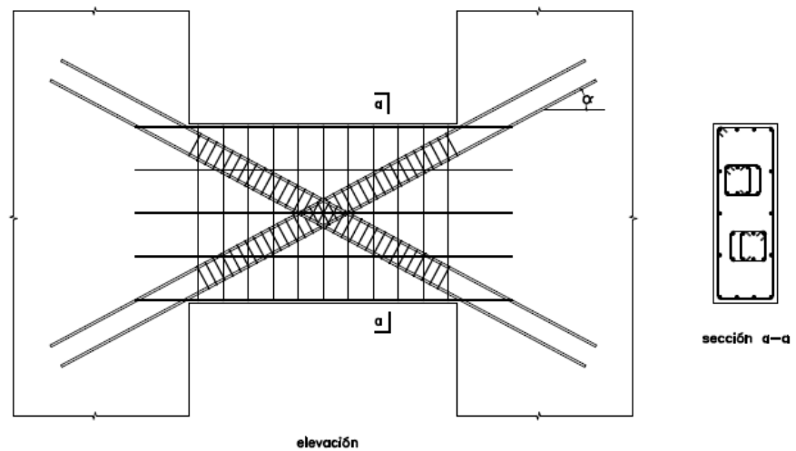
Fig. 21.9.9.5 i Refuerzo de vigas de acople.
