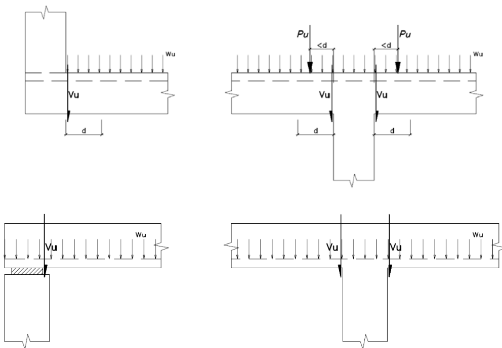
Fig. 11.1.3.1 B Condiciones de apoyo y de aplicación de las cargas externas en las cuales no se puede reducir la fuerza V_u de diseño
