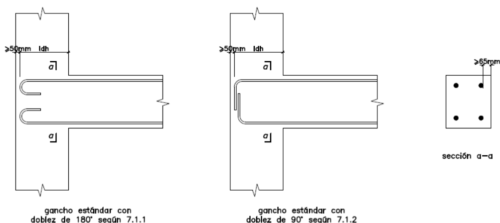
Fig. 21.5.3.a) Casos en los que se puede multiplicar l_{dg} por 0,7.
