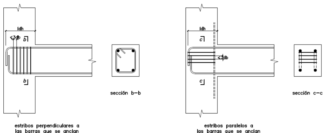
Fig. 21.5.3.b) Casos con gancho estándar a 90° en los que se puede multiplicar l_{dg} por 0,8.
