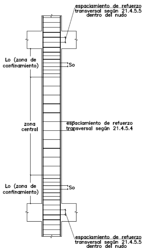
Fig. 21.4.5 Requerimientos de estribos en columnas.
