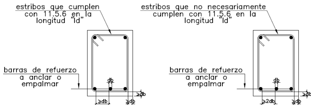
Fig. 12.1 Condiciones para la longitud de desarrollo de barras en tracción.
