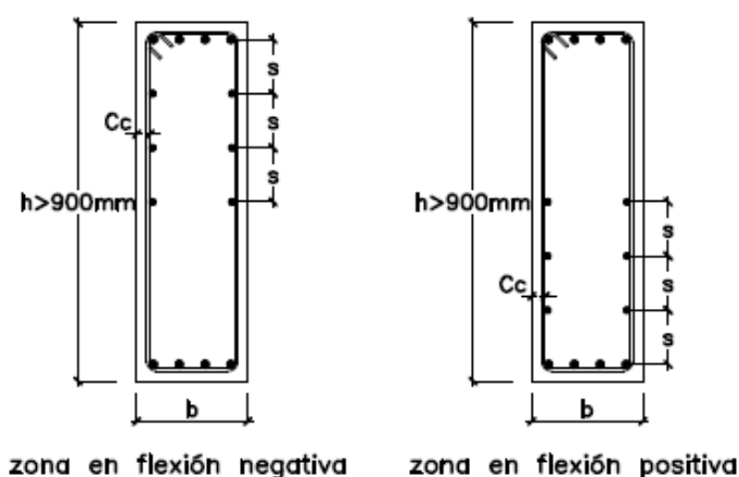
Fig. 9.9.6 Refuerzo superficial en vigas con peralte mayor a 900 mm.
