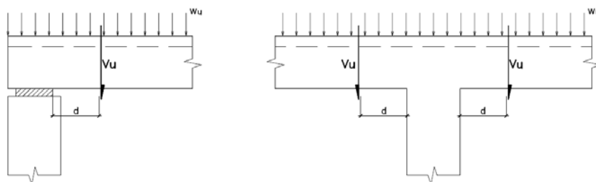
Fig. 11.1.3.1 A Condiciones de apoyo y de aplicación de las cargas externas en las cuales se puede reducir la fuerza V_u de diseño
