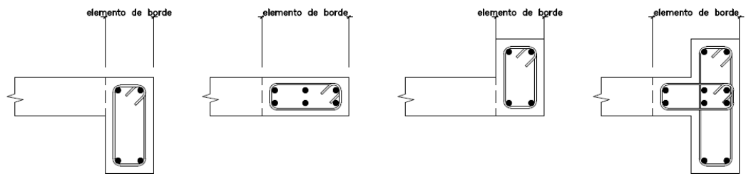
Fig. 21.1 c Ejemplos de elementos de borde en diafragmas estructurales.
