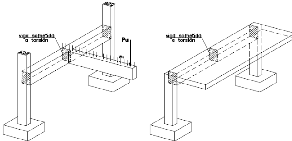
Fig. 11.6.2.1 Casos en los cuales la resistencia a la torsión afecta directamente al equilibrio de la estructura (torsión de equilibrio)
