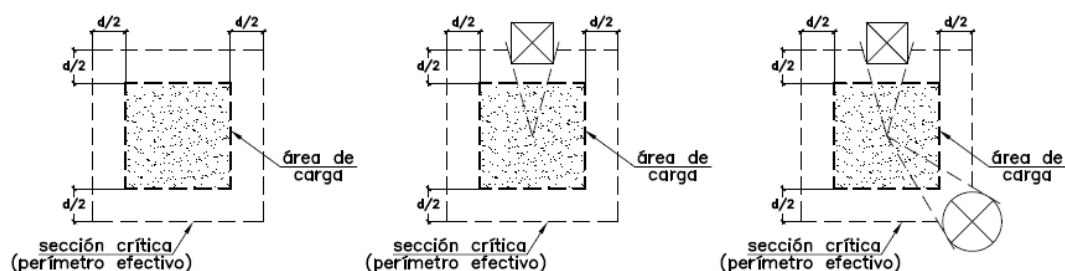
Fig. 11.12.5.1.i Aberturas en losas (las líneas discontinuas muestran el perímetro efectivo).
