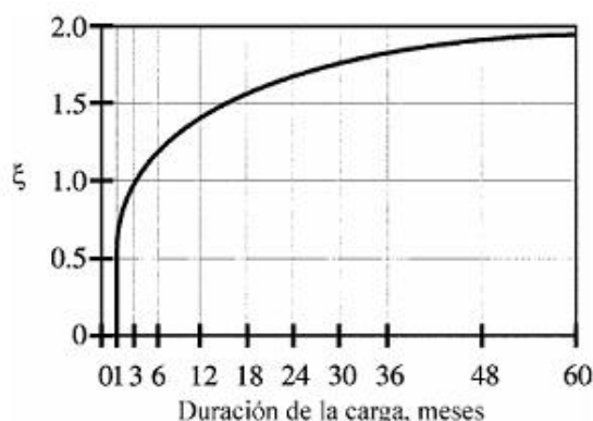
Fig. 9.6.2.5 Factor dependiente del tiempo para cargas sostenidas.
