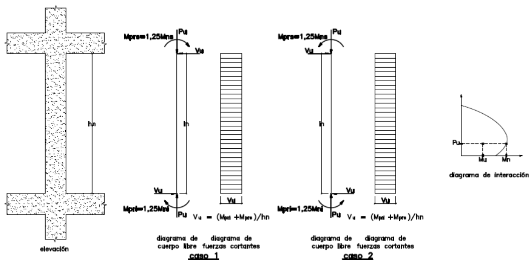
Fig. 21.6.5.1 Fuerza cortante de diseño en columnas.
