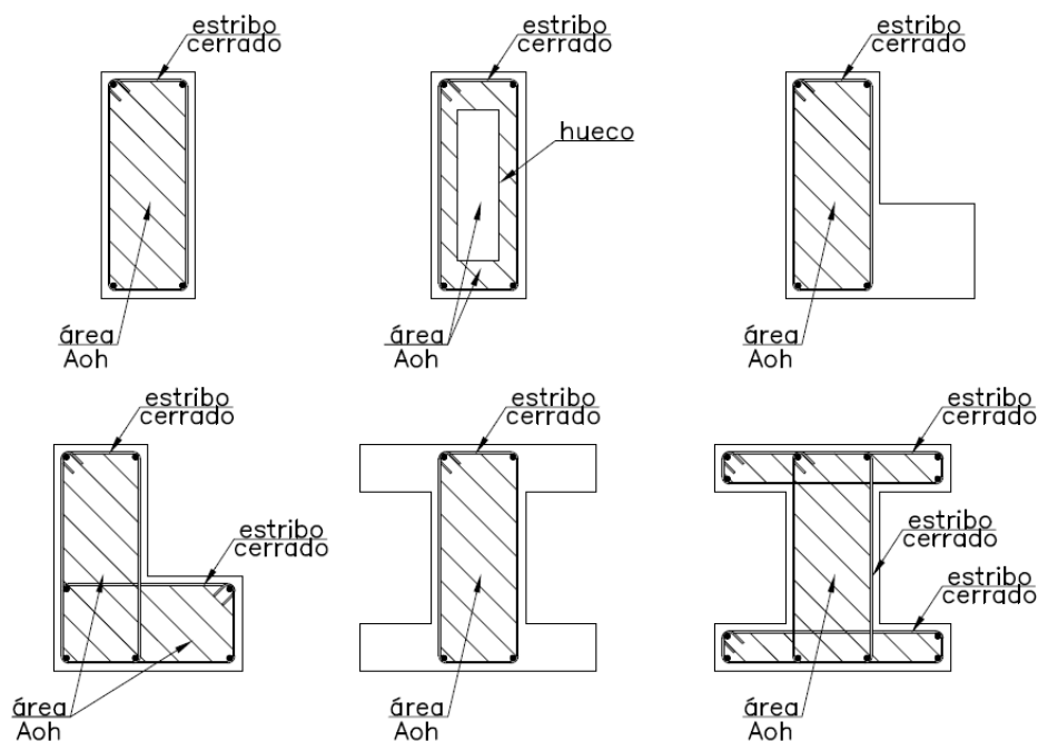
Fig. 11.6.3 Definición de A_{oh} (área sombreada)
