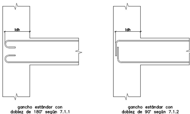
Fig. 12.5.2 Longitud de anclaje con gancho estándar en tracción.
