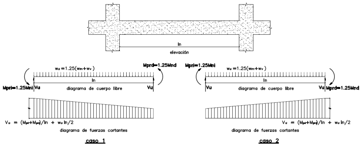
Fig. 21.5.4.1 Fuerza cortante de diseño en vigas.
