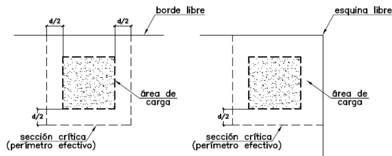
Fig. 11.12.5.1.ii Bordes libres en losas (las líneas discontinuas muestran el perímetro efectivo).
