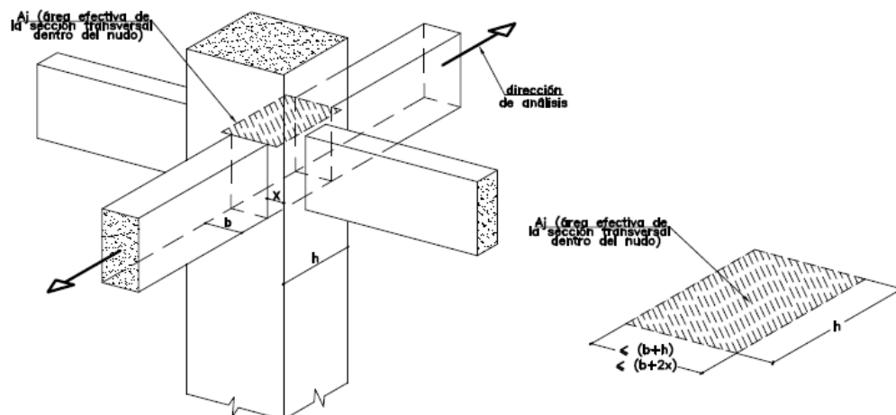
Fig. 21.7.4.1 Área efectiva en el nudo.
