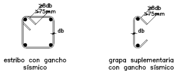
Fig. 21.1 d Ganchos sísmicos en estribos y grapas suplementarias
