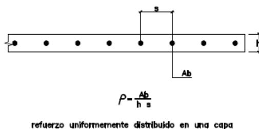
Fig. 21.10.2.8 Cuantía de acero en bordes no confinados.
