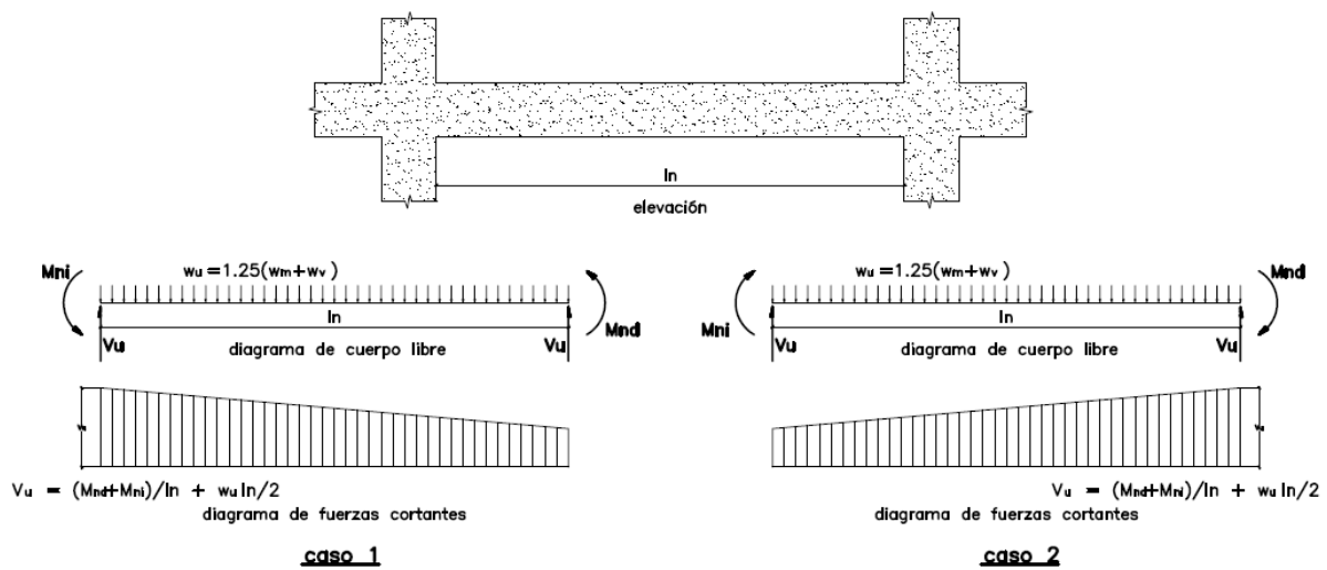
Fig. 21.4.3 i Fuerza cortante de diseño en vigas.
