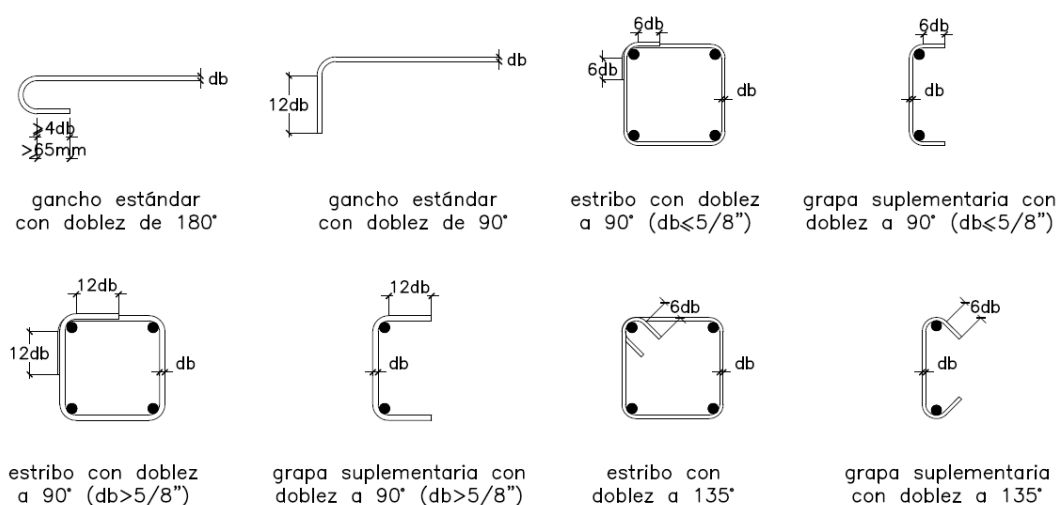
Fig. 7-1 Ganchos de barras longitudinales, estribos y grapas suplementarias.
