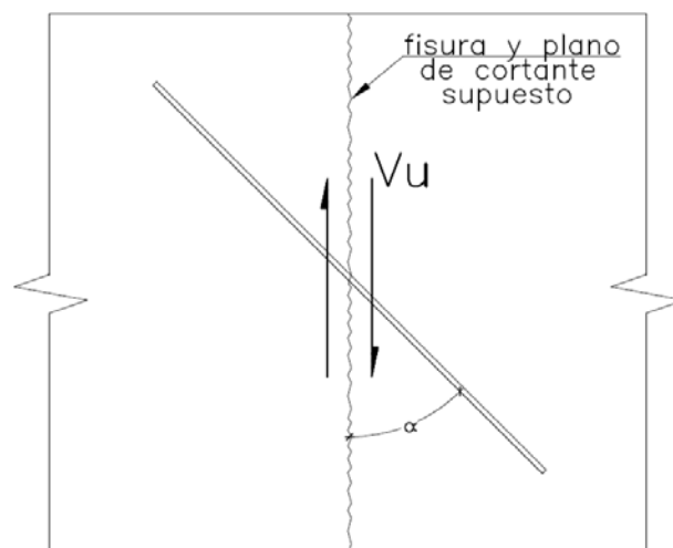
Fig. 11.7.4.2 Refuerzo de cortante por fricción inclinado con respecto a la fisura supuesta
