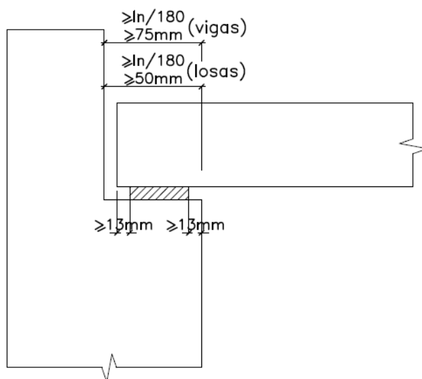
Fig. 16.6.2. Longitud de apoyo de un elemento prefabricado.
