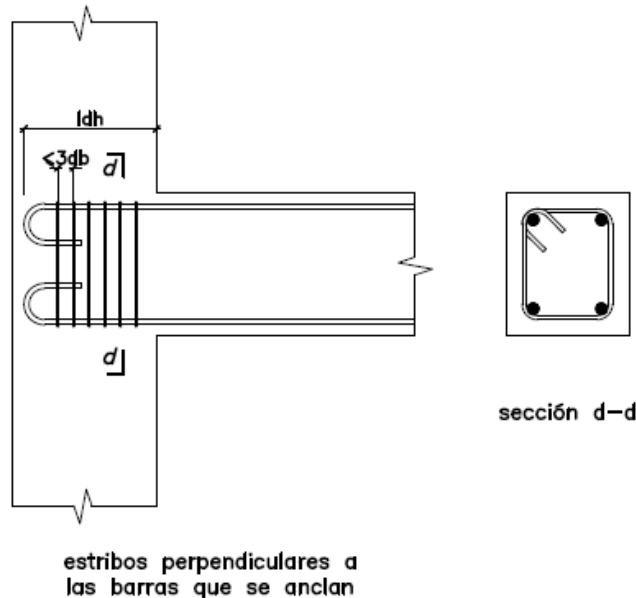
Fig. 21.5.3.c) Caso con gancho estándar a 180° en el que se puede multiplicar l_{dg} por 0,8.
