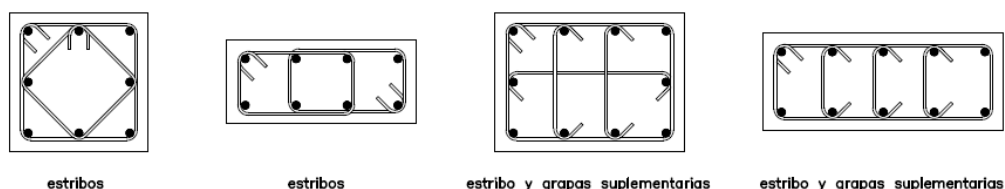
Fig. 21.1 a Ejemplos de configuraciones de los estribos de confinamiento.
