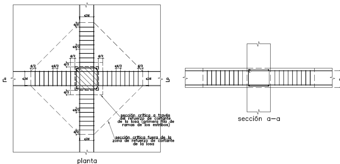
Fig. 11.12.3.i Disposición de los estribos por cortante en columnas interiores.
