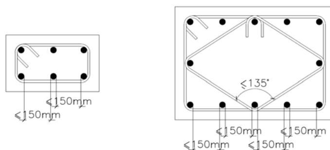
Fig. 7.10.5.3 Separación máxima de barras sin apoyo lateral.
