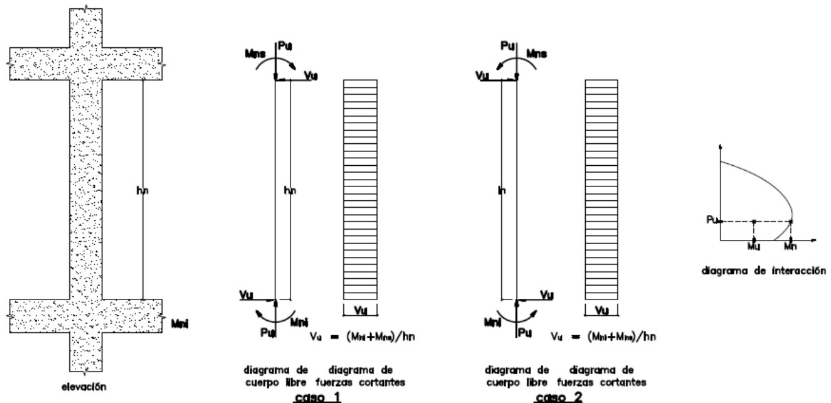
Fig. 21.4.3 ii Fuerza cortante de diseño en columnas.
