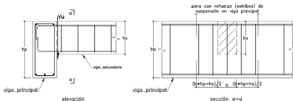
Fig. 11.5.8 Refuerzo de suspensión
