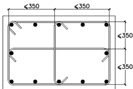
Fig. 21.6.4.3 Distancia máxima entre ramas del refuerzo transversal.
