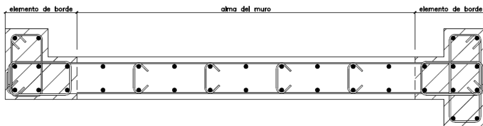
Fig. 21.1 b Ejemplo de elementos de borde en muros.
