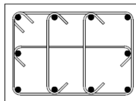
1 estribo y 3 grapas suplementarias
