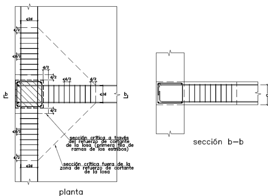
Fig. 11.12.3.ii Disposición de los estribos por cortante en columnas de borde.
