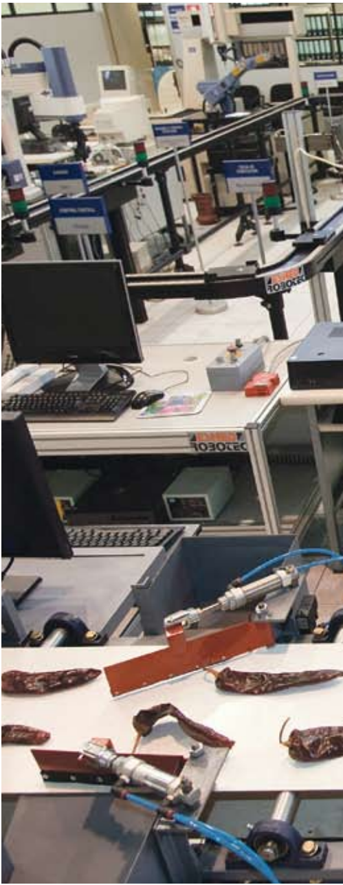
TECNOLOGÍA DE PUNTA. Módulo mecánico donde se clasifican las paprikas. En la foto se aprecia cómo se clasifica la
